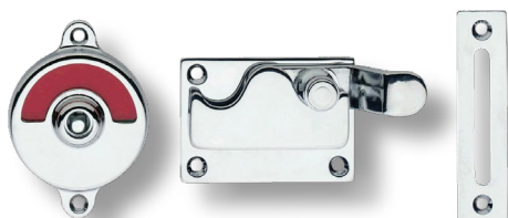
Toiletlås – Forkrøbbet rigle Finish: Blank krom Vare nr.: 0016.370001
